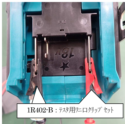
図 1-3 ワニクリップ取付
