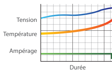
Charge conventionnelle
